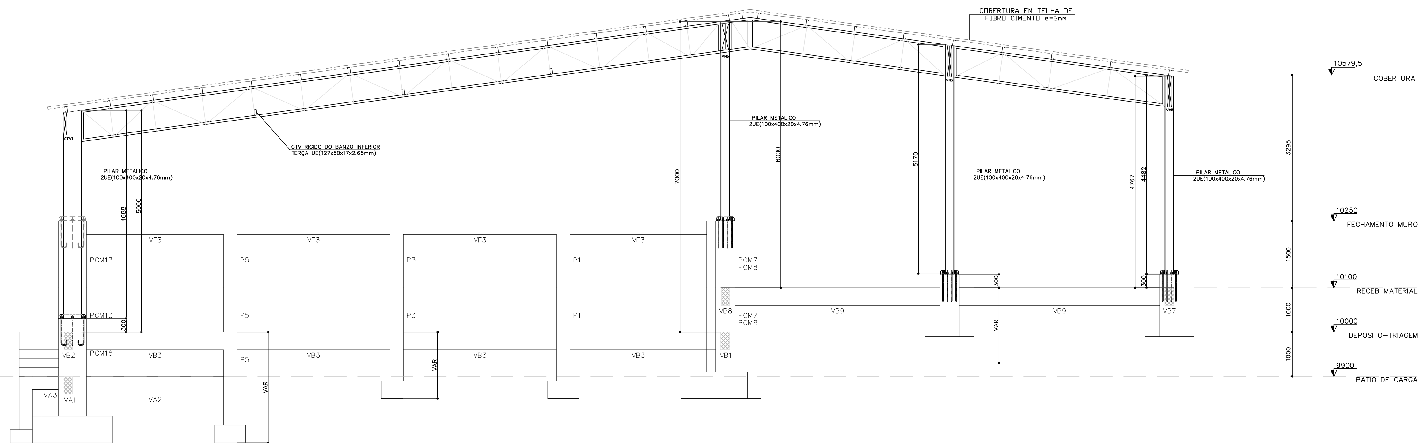
COORTE B-B ESCALA 1:50
